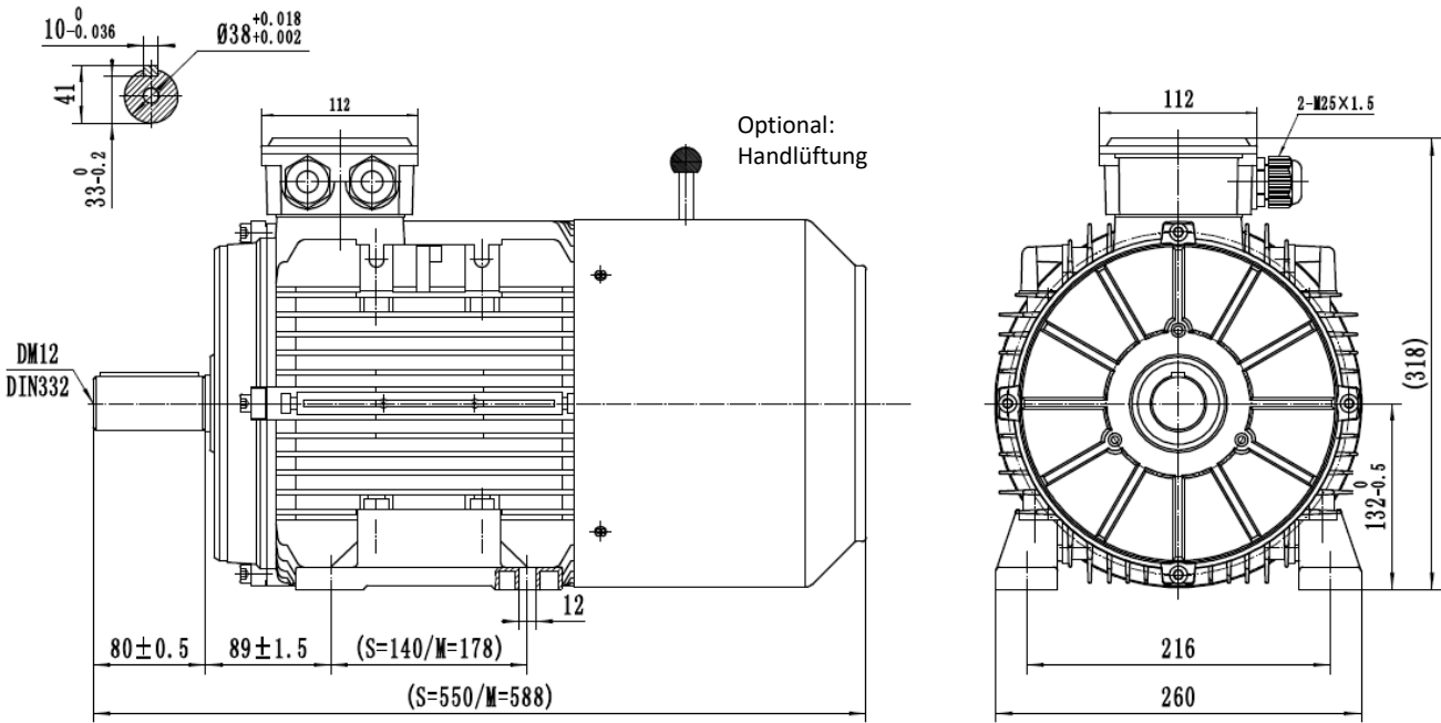
Typ / type SEV-BM3 132M1-4
