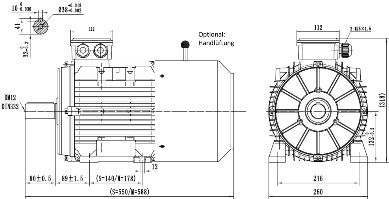
Typ / type SEV-BM3 132S-4
