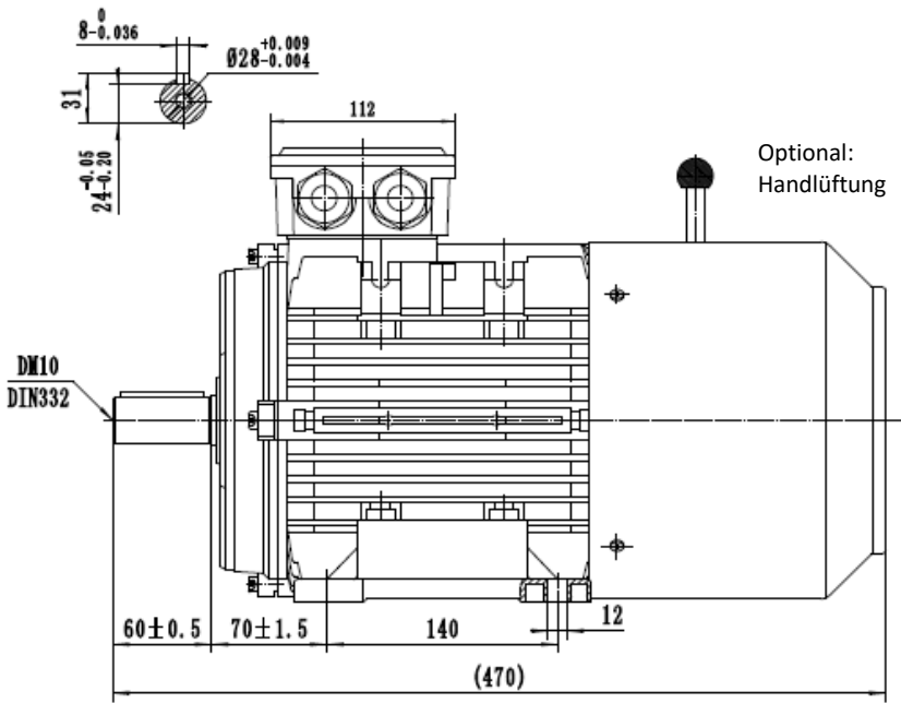
Typ / type SEV-BM3 112M1-4
